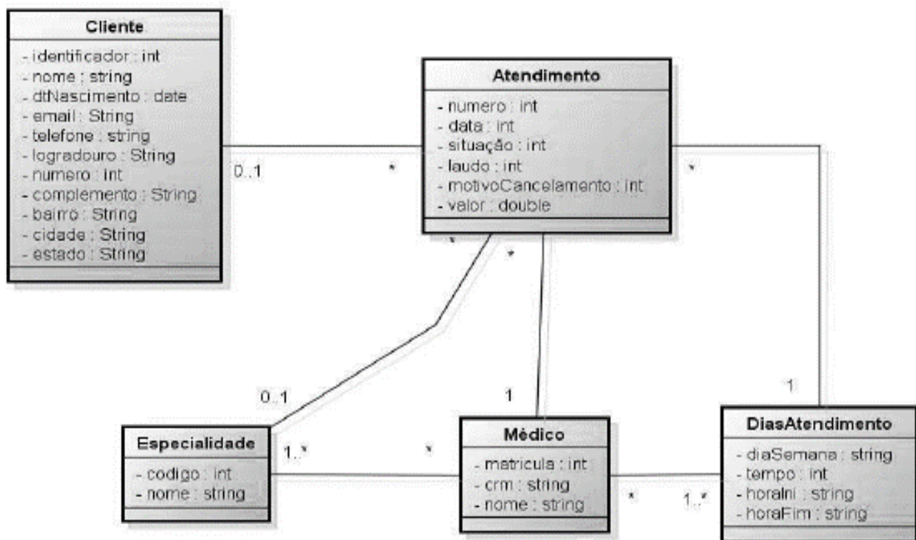
Figura 6 - Diagrama de Classes
