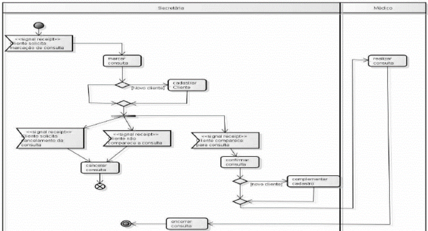
Figura 5 - Diagrama de Atividades
